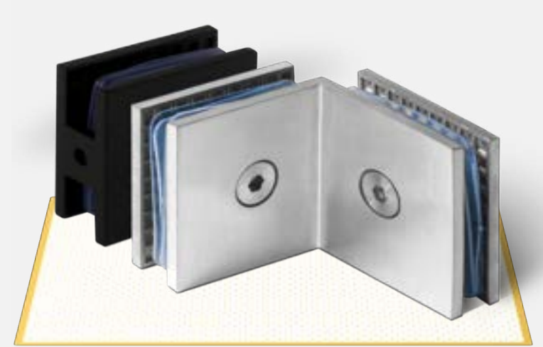
3 Fix üveg megfogók
