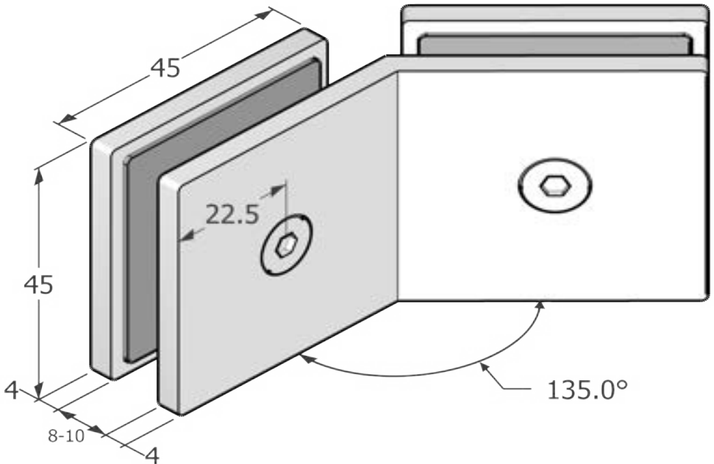
Sarok fix megfogó üveg/üveg, 135° 8-12 mm AISI304
