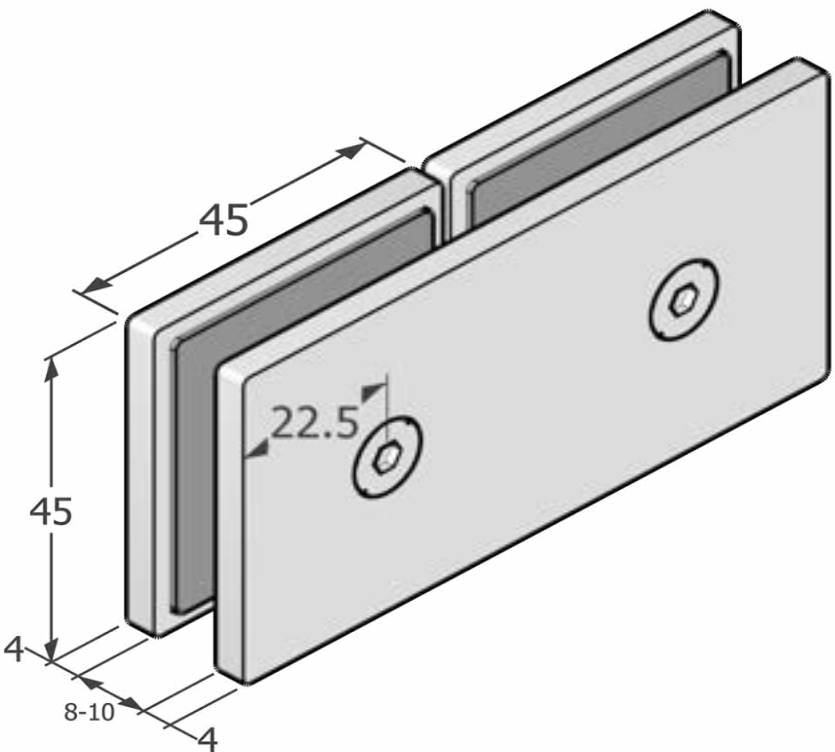
Fix megfogó üveg/üveg, 180° 8-12 mm AISI304
